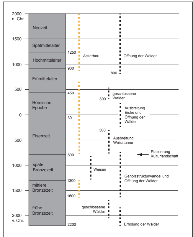
Abb. 10: Übersicht über die regionale Waldentwicklung am Obersee.
